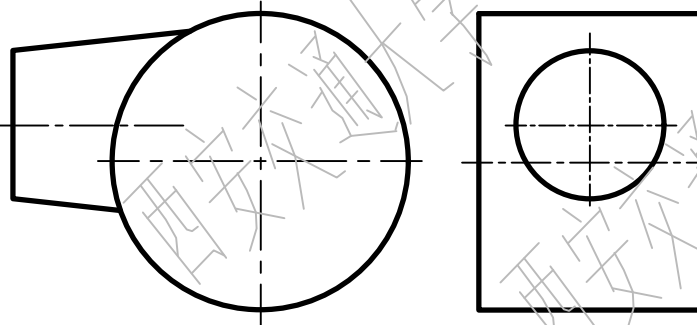
4-30 画出俯视图，补全左视图，标出特殊点，并保留必要的辅助线。
