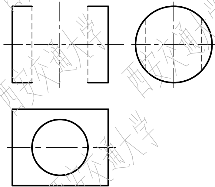
4-26 画出主视图。
