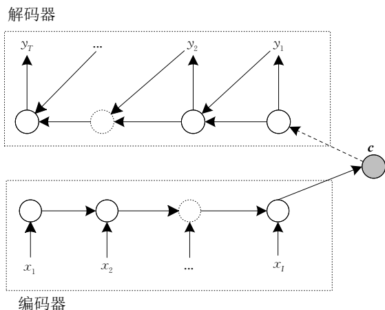
图 2 编码器解码器模型
