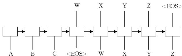
图 1 端到端模型
