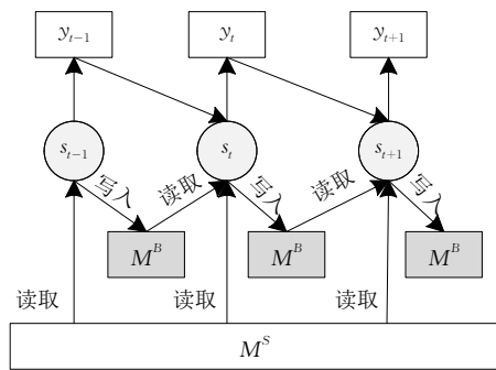
图 6 MEMDEC 解码方法图示
