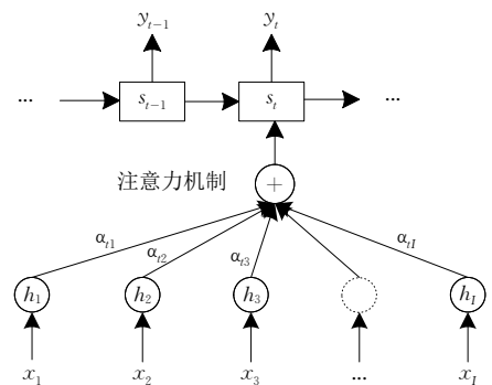
图 5 注意力机制图示
